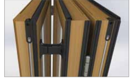
Sicherheitsfunktionsschnapper zur Feststellung des Drehflügels panel catcher for additional security to fix the pass door to the adjacent panel
